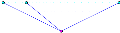
Bild 1: \mathcal{T}(\tilde{\Gamma}_{1,t}^\circ)
